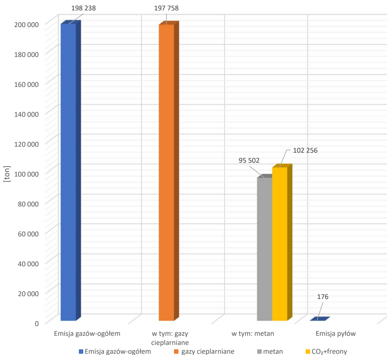
Wykres 4. Emisja gazów i pyłów do powietrza atmosferycznego w okresie I kwartału 2023 r.
