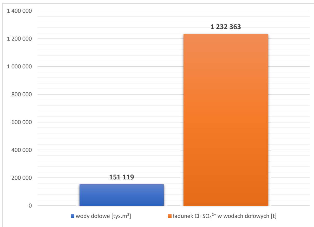
Wykres 3. Ilość wód dołowych odprowadzonych oraz ładunek soli w odprowadzonych wodach w okresie 3 kwartałów 2024 r.
