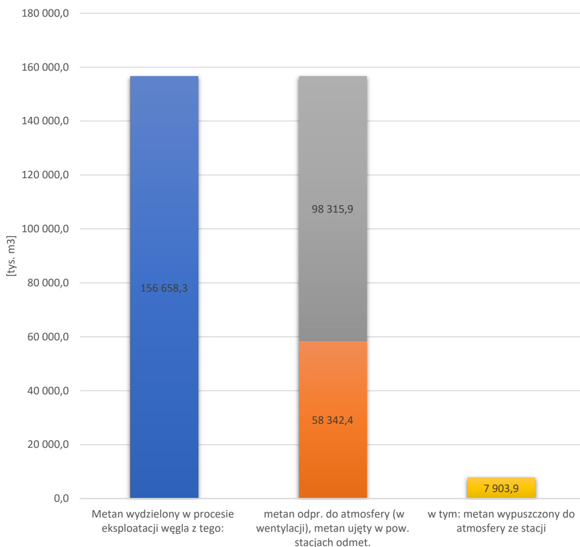
Wykres 2. Wydzielenie, ujęcie oraz emisja metanu do atmosfery w okresie I kwartału 2025 r.
