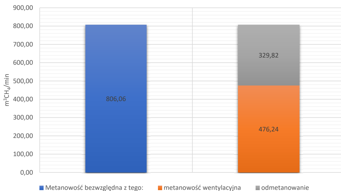
Wykres 1. Metanowość eksploatowanych ścian w kopalniach węgla kamiennego w okresie I kwartału 2025 r.
