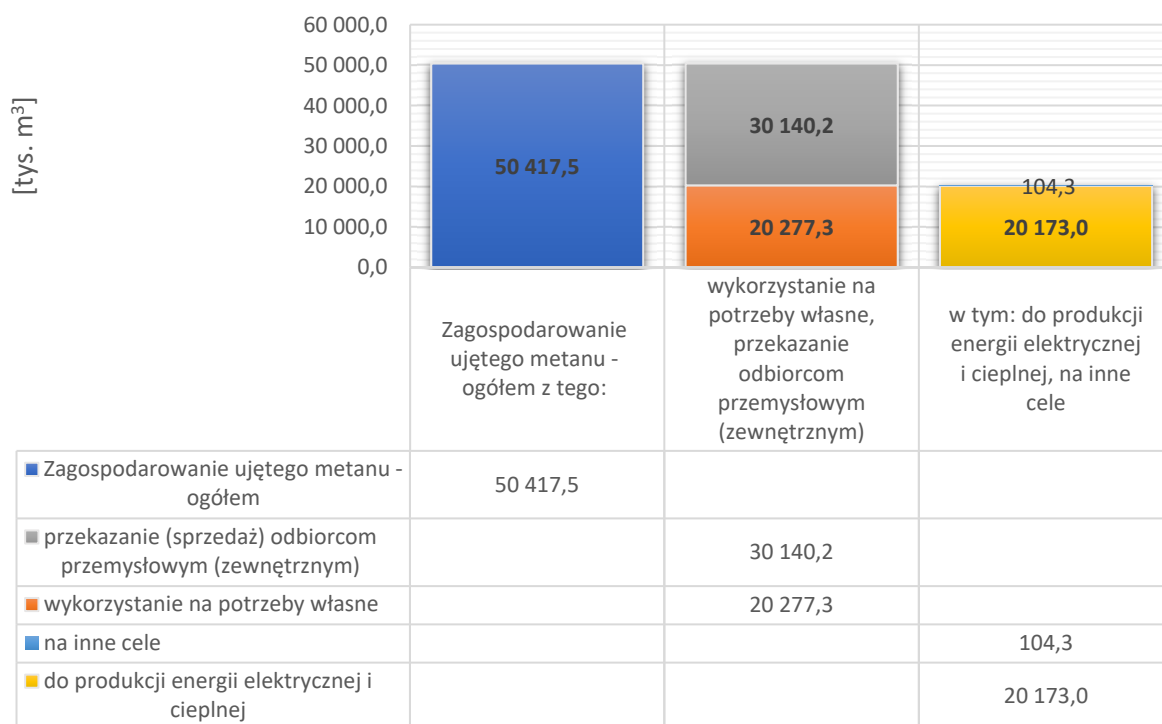
Wykres 3. Zagospodarowanie ujętego metanu w okresie I kwartału 2025 r.
